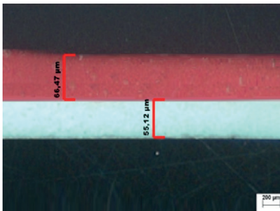
metallografische dwarsdoorsneden
